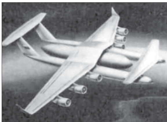
Проектный эскиз транспортного самолета «Геракл»
