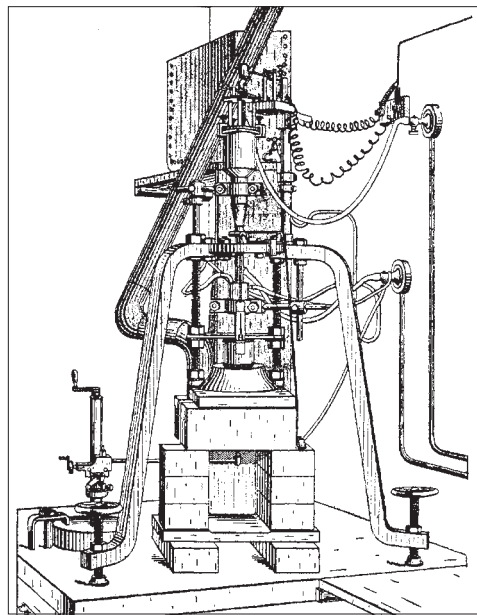
Схема печи Вернейля
