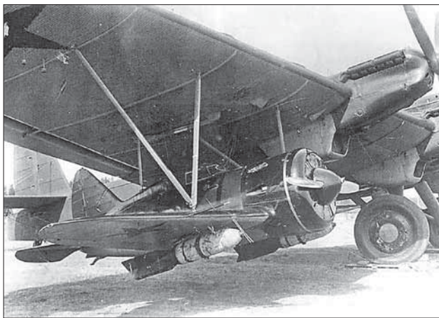
Истребитель И-16 под крылом бомбардировщика ТБ-3
