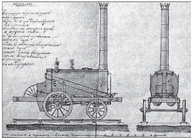
Примерно так выглядел паровоз Черепановых
