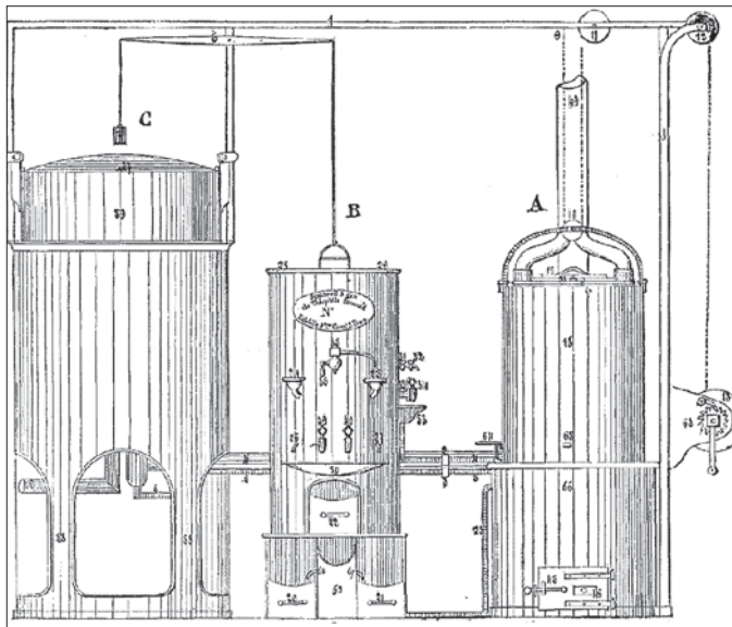
Схема установки для производства светильного газа
