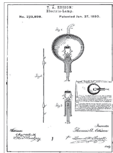
Патент, выданный Эдисону на электролампочку
