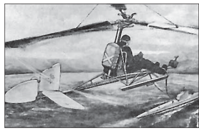
Немецкий воздушный змей-автожир «Фокке — Анхелис Fa-330A»
